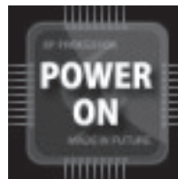
起動画面
