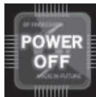
終了画面
